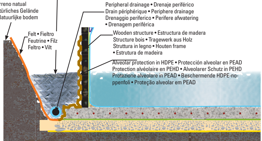
Alveolar protection in HDPE Protección alveolar en PEAD Protection alvéolaire en PEHD Alveolar Schutz in PEHD Protezione alveolare in PEAD Beschermdende HDPE-noppenfoli Proteção alveolar em PEAD
